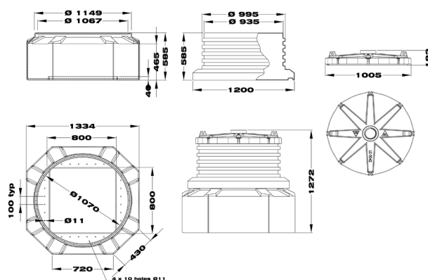
Chambre de visite étanche, polyéthylène, modèle profond.
