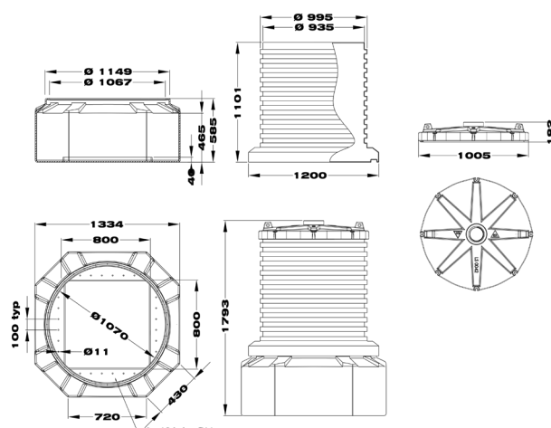
Chambre de visite étanche, polyéthylène, modèle profond, avec réhausse allongée.
